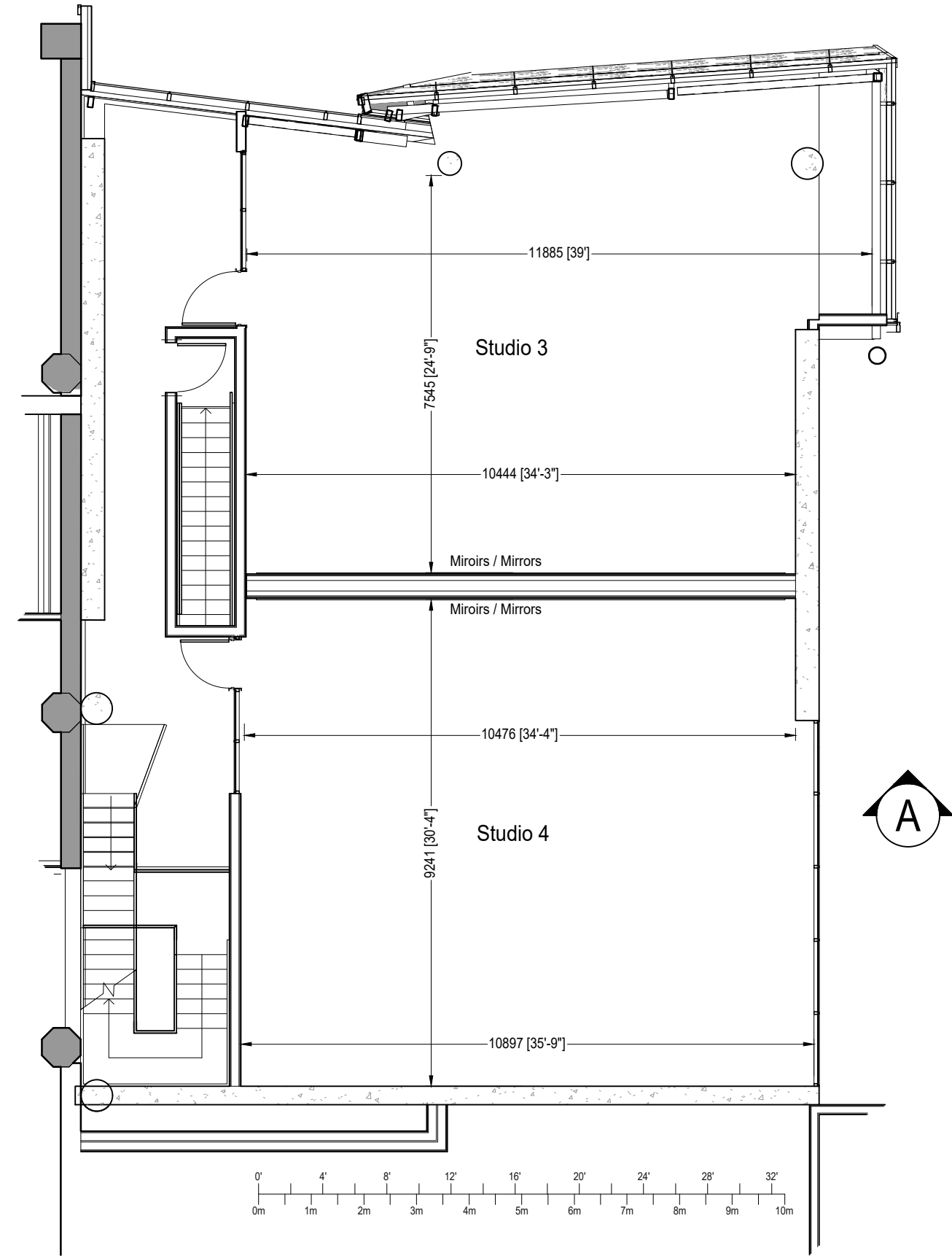
Plan 3e Étage Plan 3rd Level
